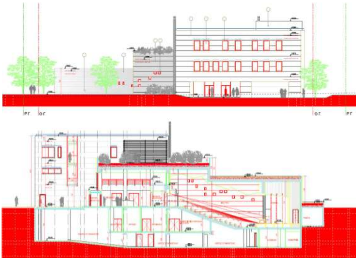
Όψη και τομή του κτηρίου
