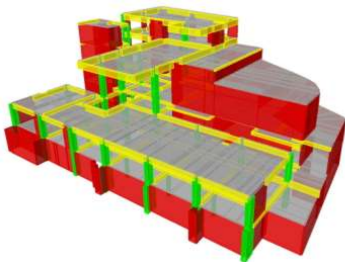
Στατικό προσομοίωμα του κτηρίου
